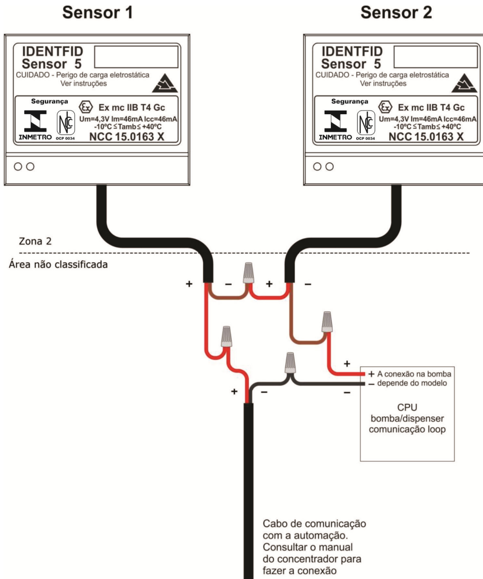
Figura 1 – Ligações IDF05
